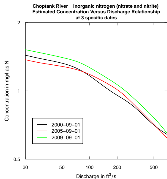
(b) plotConcQSmooth(logScale=TRUE)
